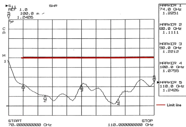
VSWR
